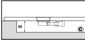
installazione in appoggio free standing shower tray
